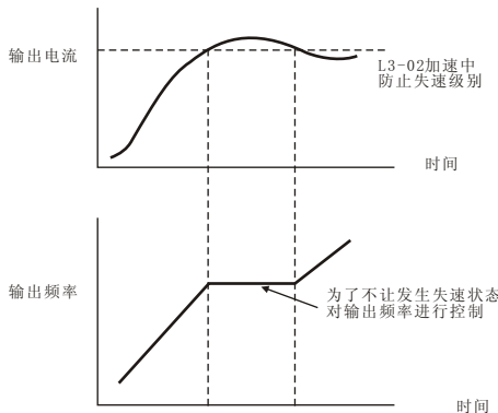
加速中失速防止功能 (L3-01=1的场合)
