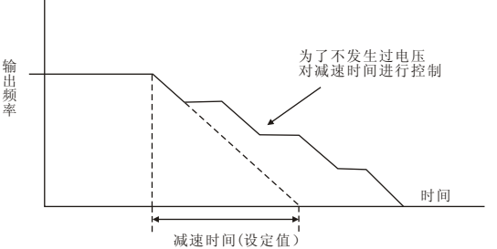
减速中失速防止动作 (L3-04=1 的场合)
